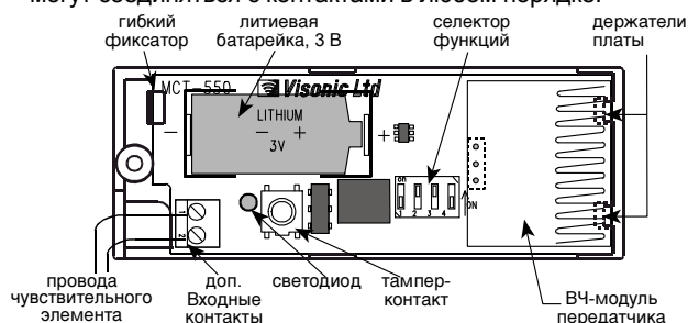
Рис. 11 - Плата
