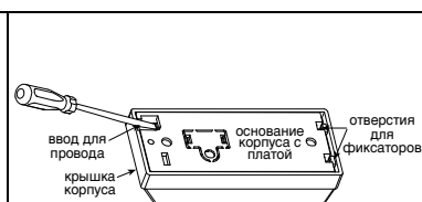
Рис. 9 - Отсоединение крышки корпуса от основания
