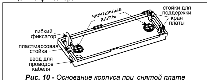
Рис. 10 - Основание корпуса при снятой плате
