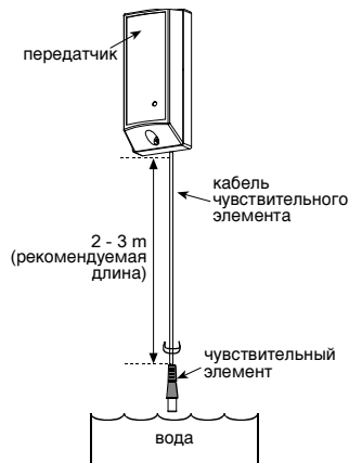
Рис. 7 - Монтаж детектора протечки
