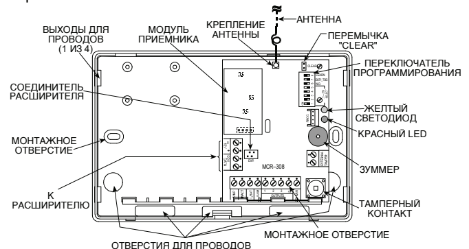
Рисунок 2. Интерфейс MCR-308 со снятой крышкой.
